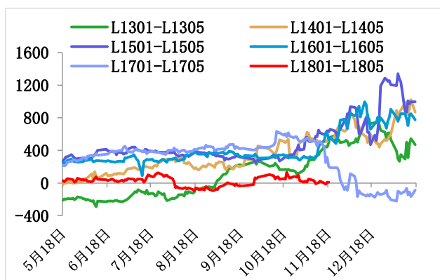
图 3：塑料 1801 合约与塑料 1805 合约价差
