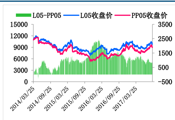
图 6：L05 合约与 PP 05 合约收盘价及价差
