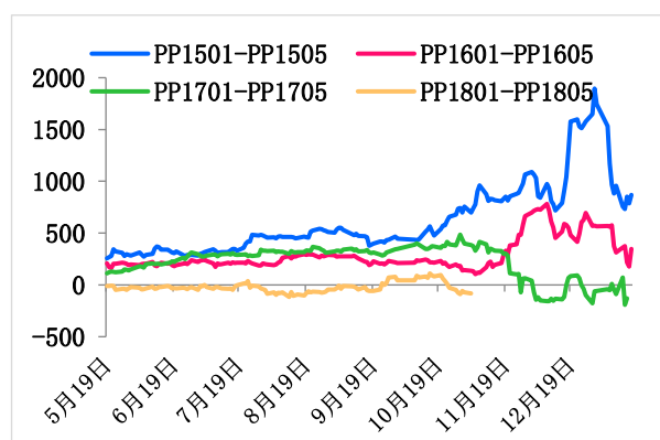
图 4：PP 1801 合约与 PP 1805 合约价差
