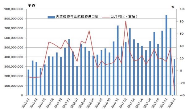
图6：天然橡胶与合成橡胶进口量
