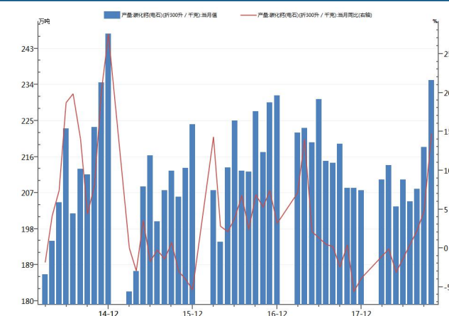
图 6：电石月度产量
