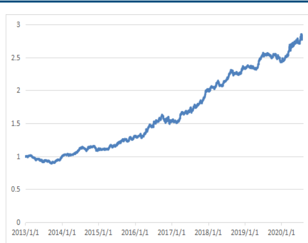
图 10：供需类策略 累计净值表现
