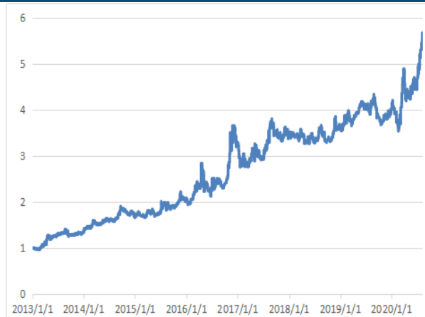
图 4：技术类策略-动量 累计净值表现
