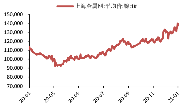
图 2: 现货镍均价
